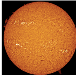
6562.8Å
